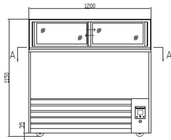
BACK 后视图
