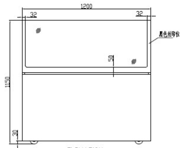
ELEVATION 前视图
